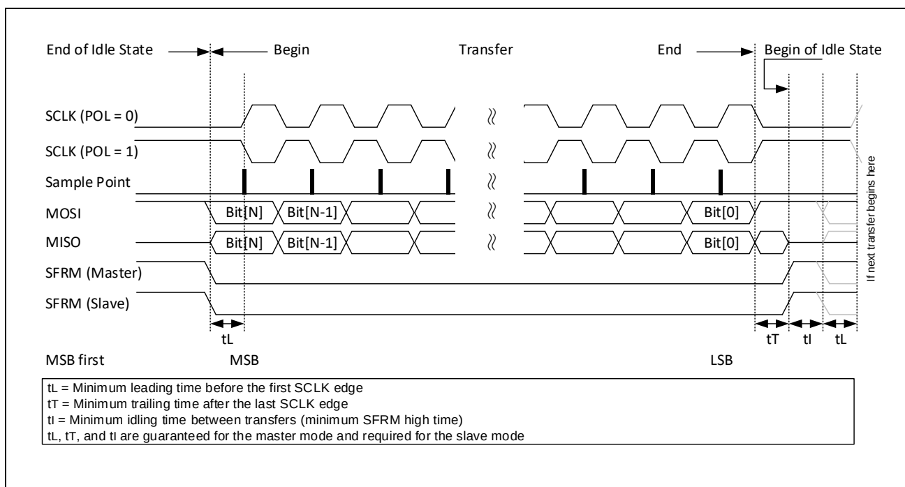
图 19-4: SSP 时钟格式 0 (PHS = 0)
