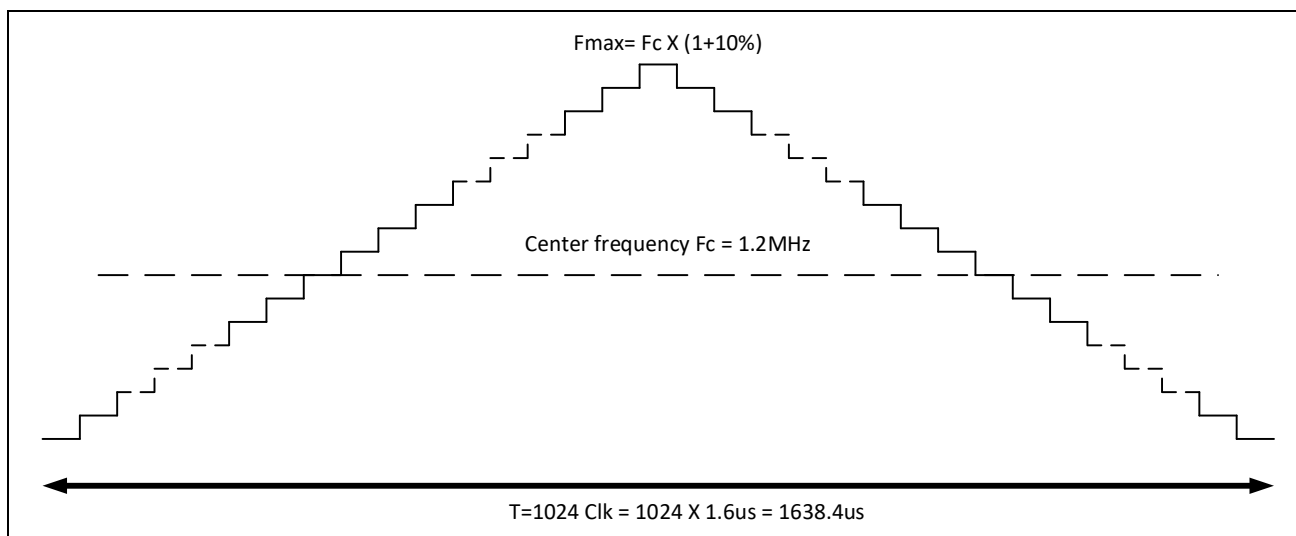
图 25-3: LV_buck 中频率抖动行为
