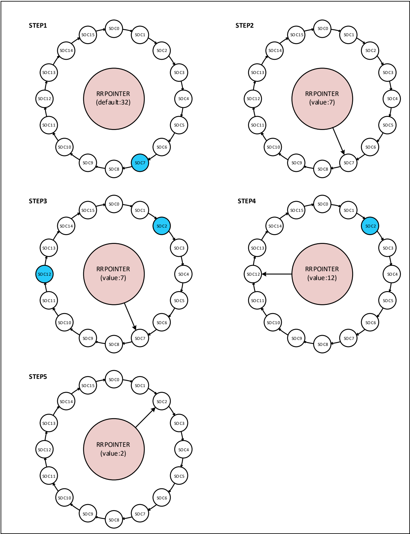
图 12-7：Round-Robin 环优先级示例
