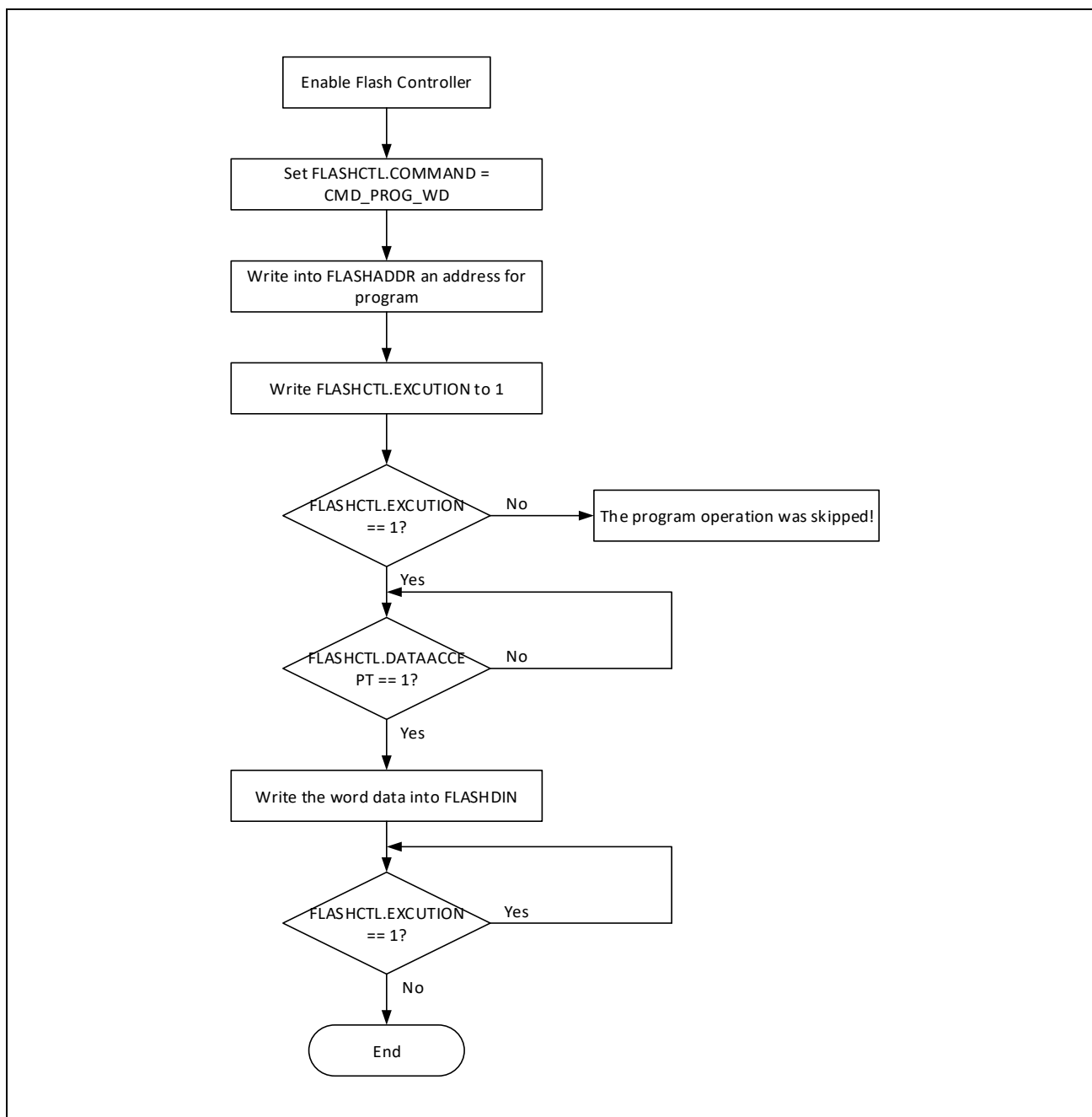
图 20-4: Flash 存储器编程操作流程
