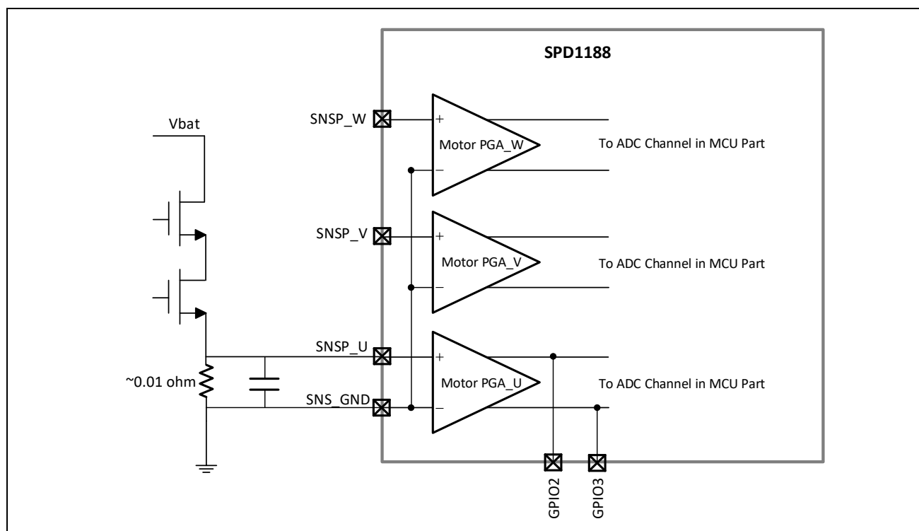
图 27-1：电机 PGA 典型应用
