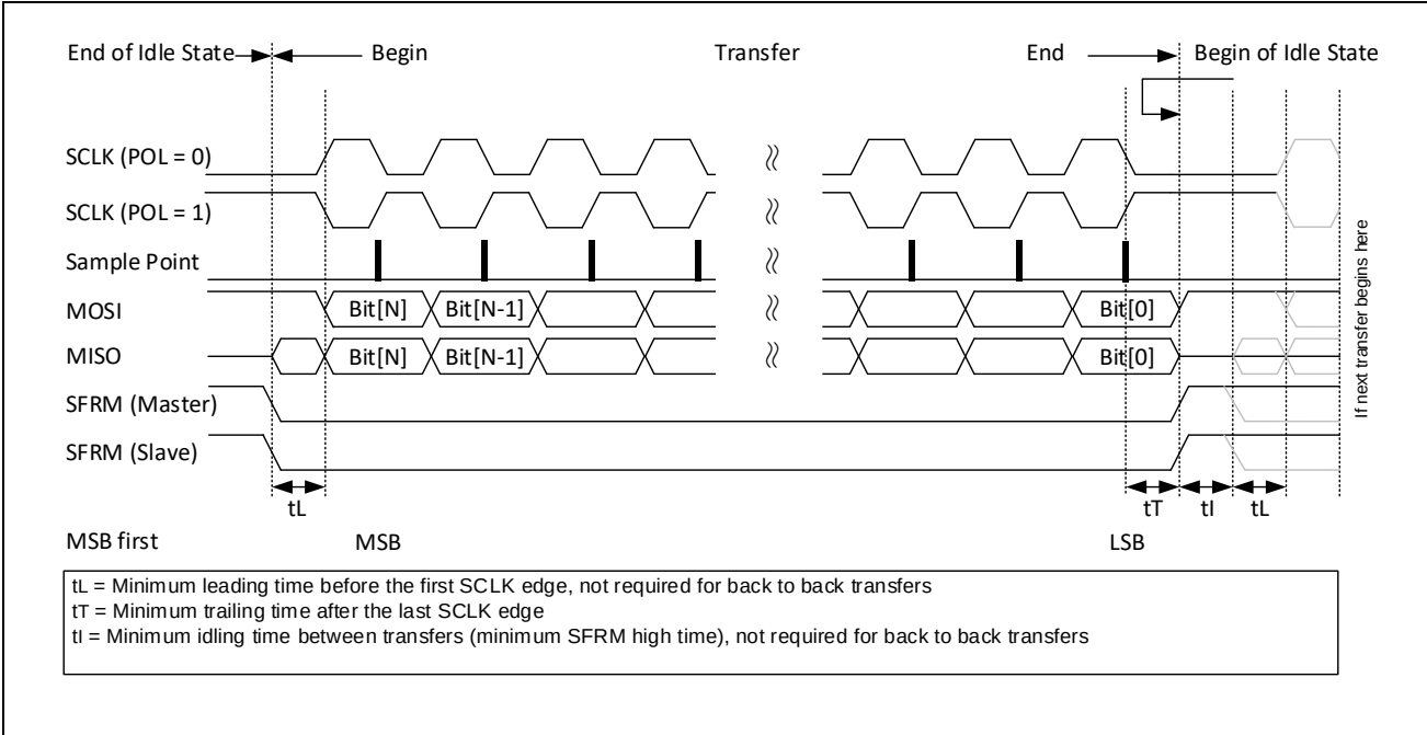
图 19-5: SSP 时钟格式 1 (PHS = 1)
