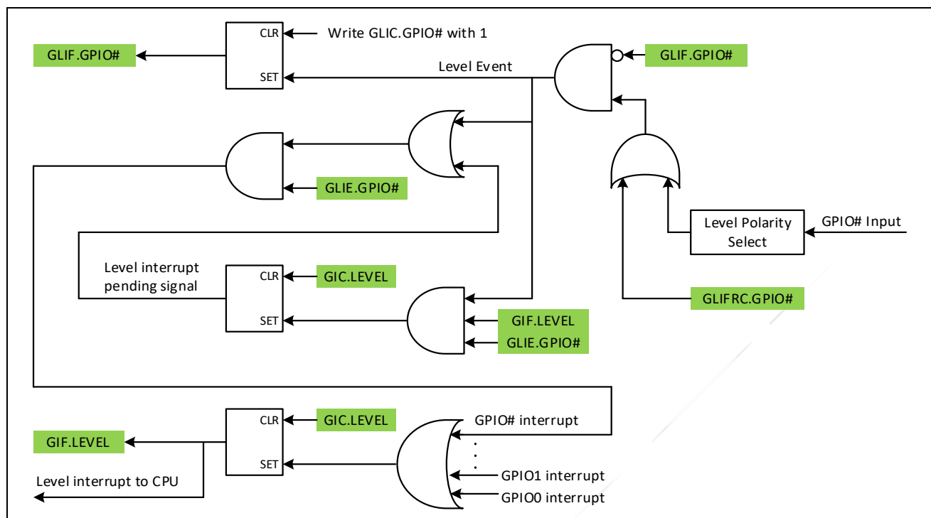
图 4-7: GPIO 电平触发中断
