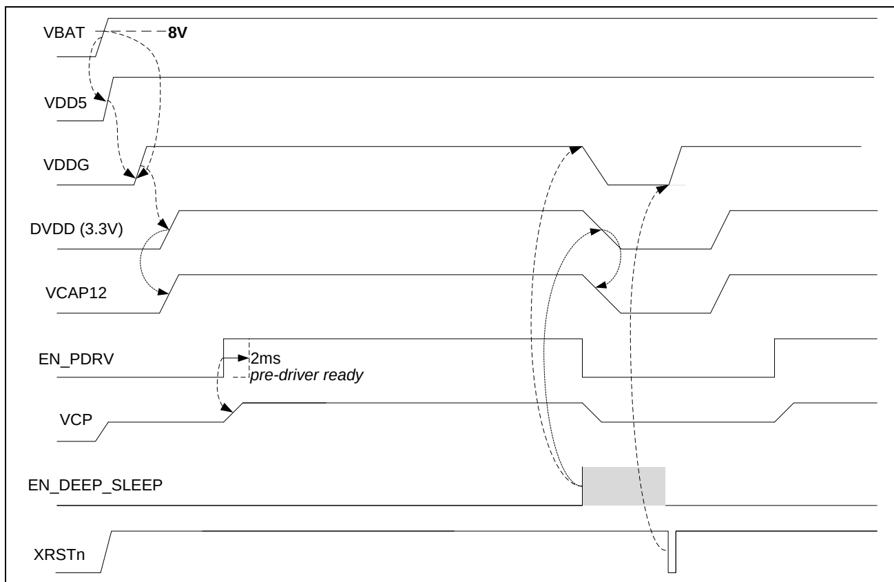
图 26-1：预驱信号上电方案
