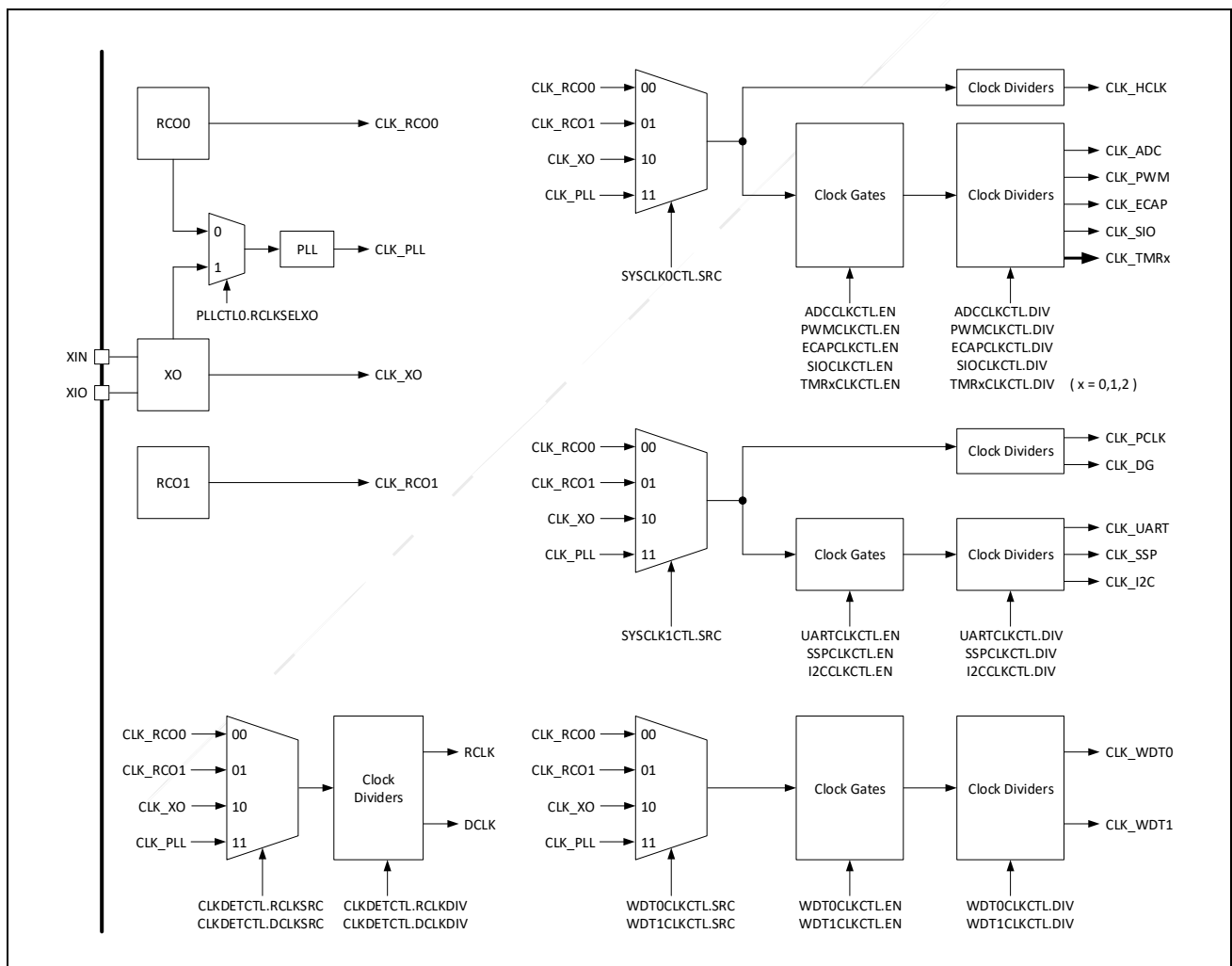
图 1-3：SPD1188 时钟树
