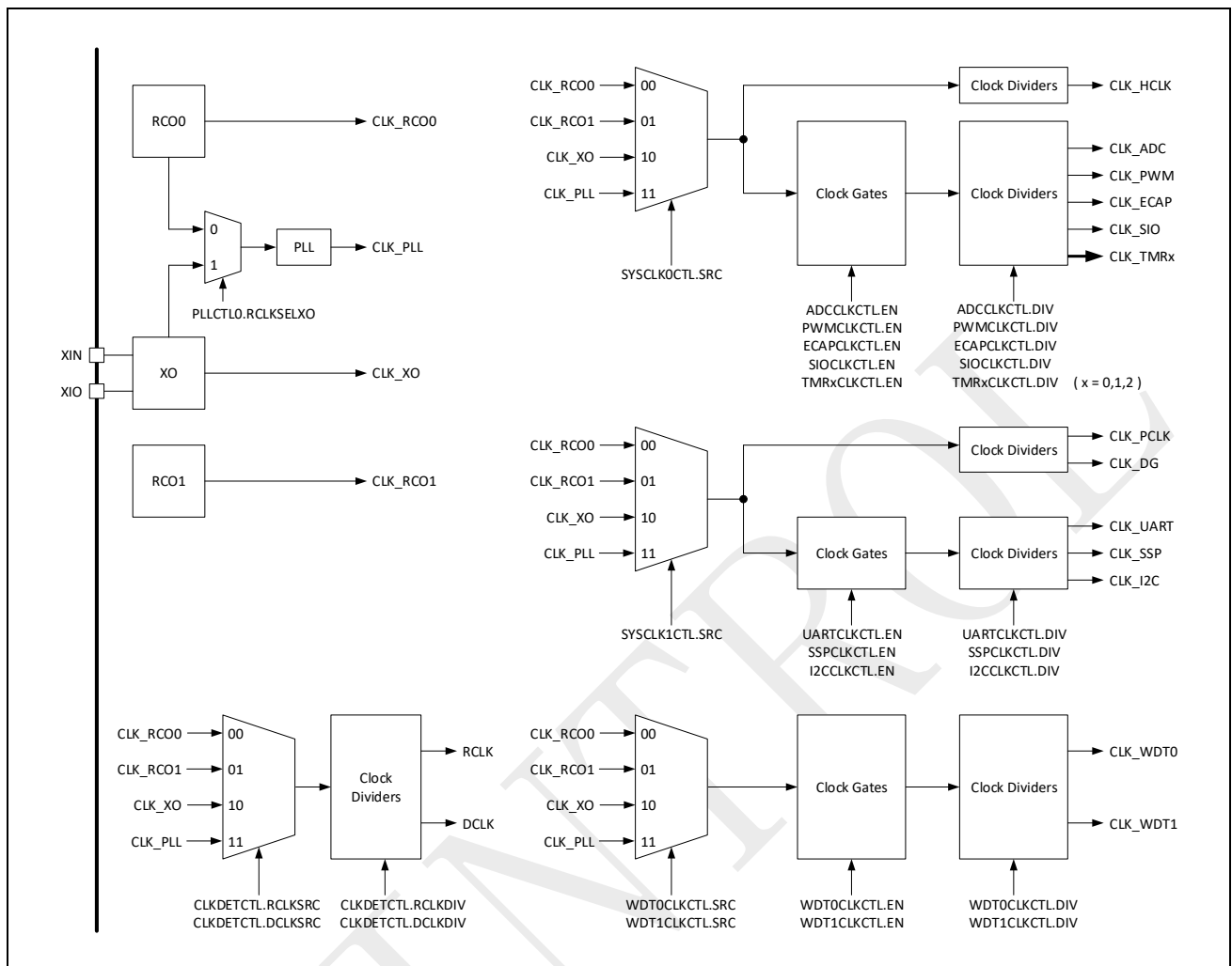
图 3-3: 时钟结构图
