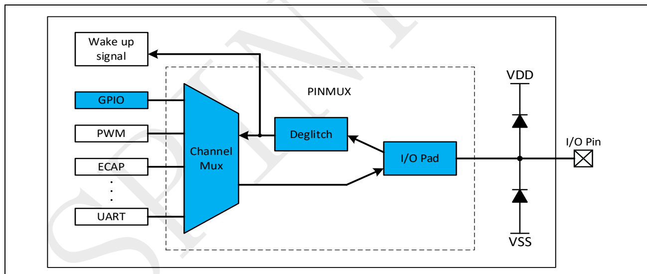
图 4-1：I/O 控制结构框图
