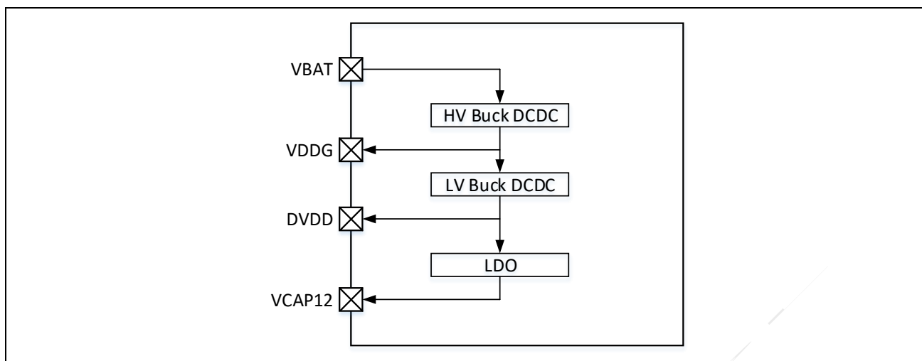
图 2-2：电源产生单元
