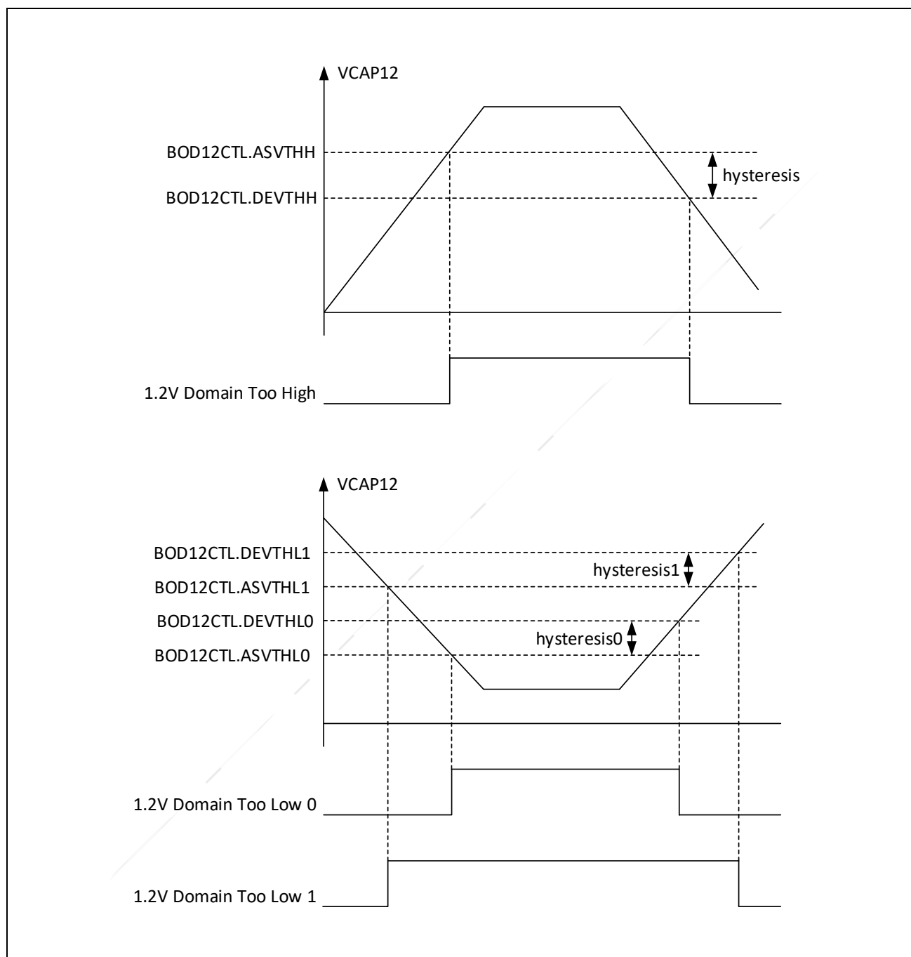
图 2-6: VCAP12 阈值
