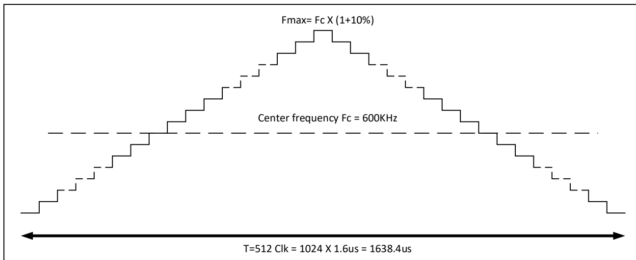
图 25-1: HV_buck 频率抖动行为
