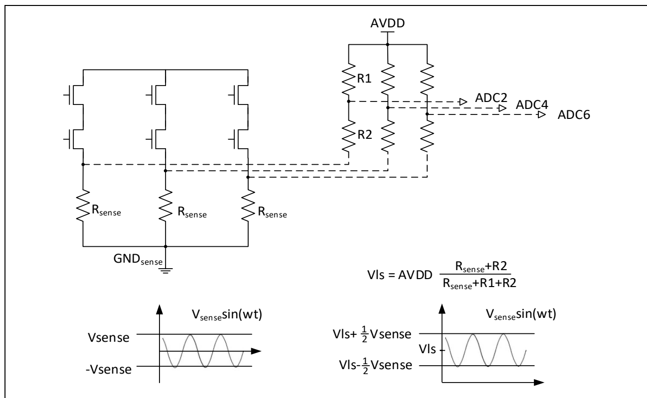
图 14-3：单端模式下采样电流示意图
