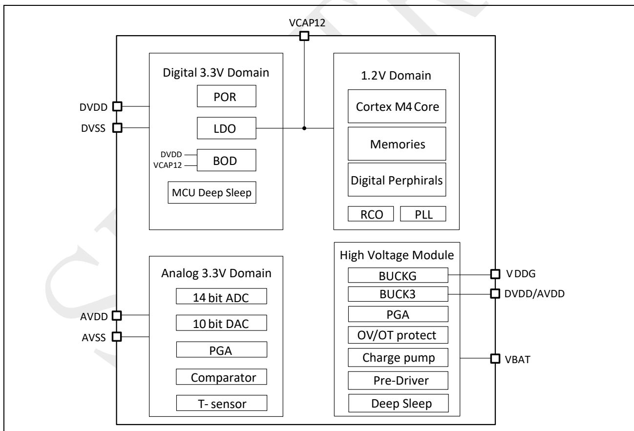
图 2-1: 电源系统总览
