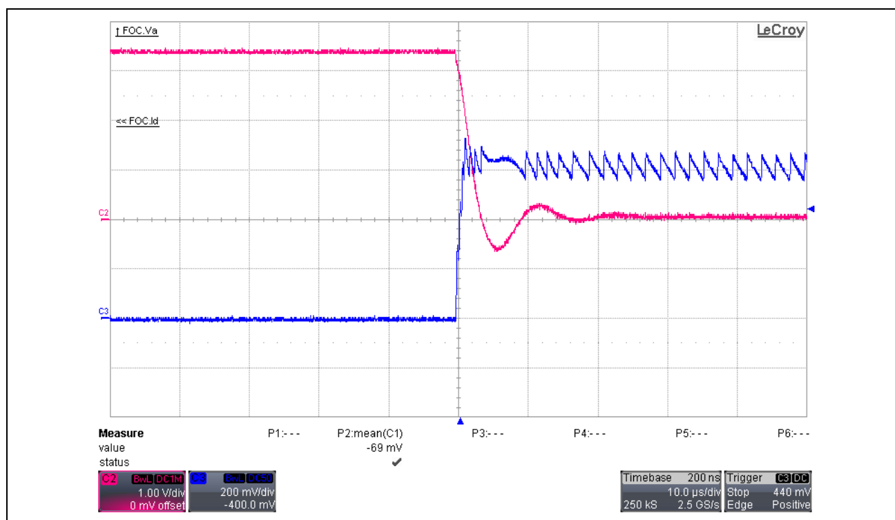
图 25-2：电流限制
