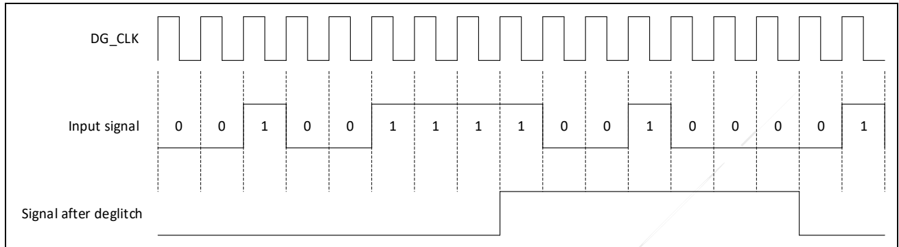
图 4-4：输入消抖
