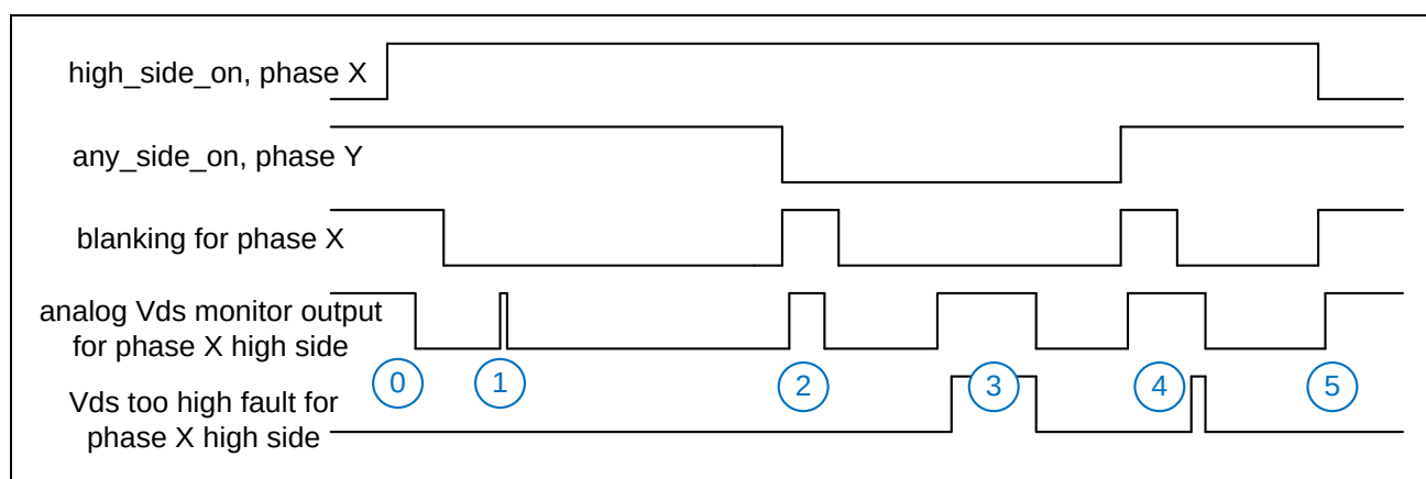
图 26-5: V_{ds} 监测器消隐框图
