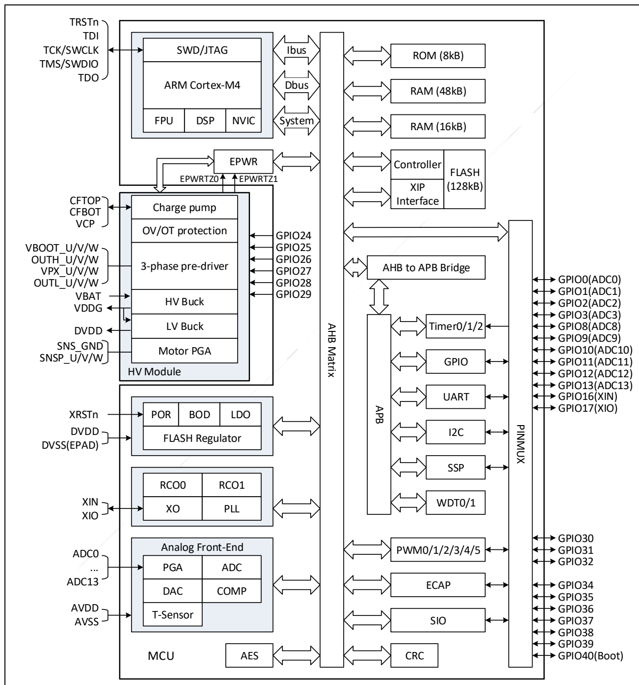
图 1-1: SPD1188 系统框图
