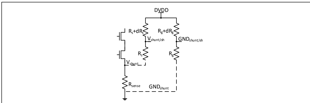
图 14-9：电平移位器电阻失配
