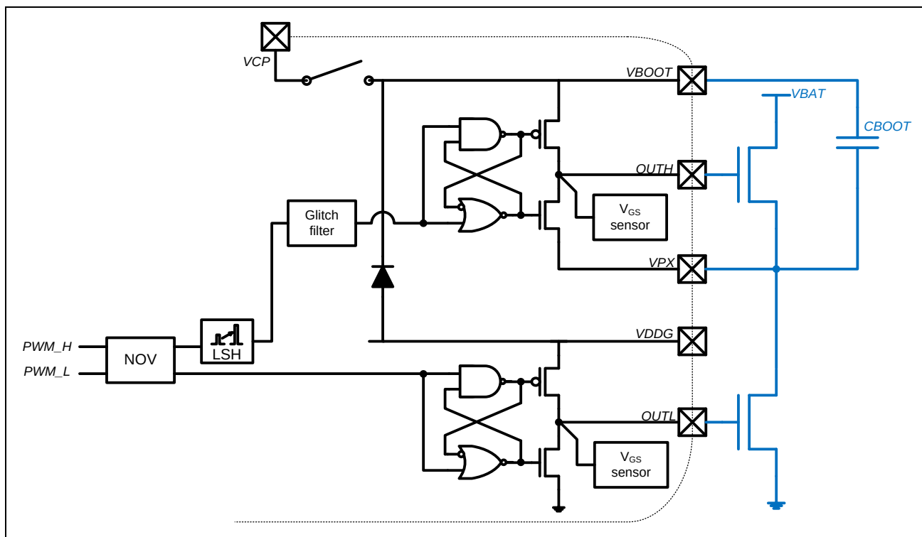
图 26-2：单相预驱简化框图
