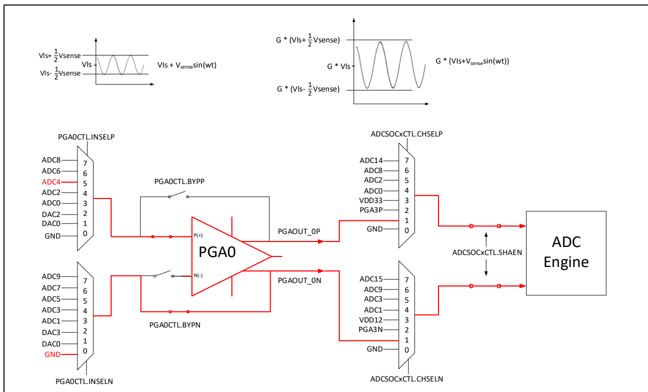
图 14-4: PGA0 选择 ADC4 作为输入（单端模式）
