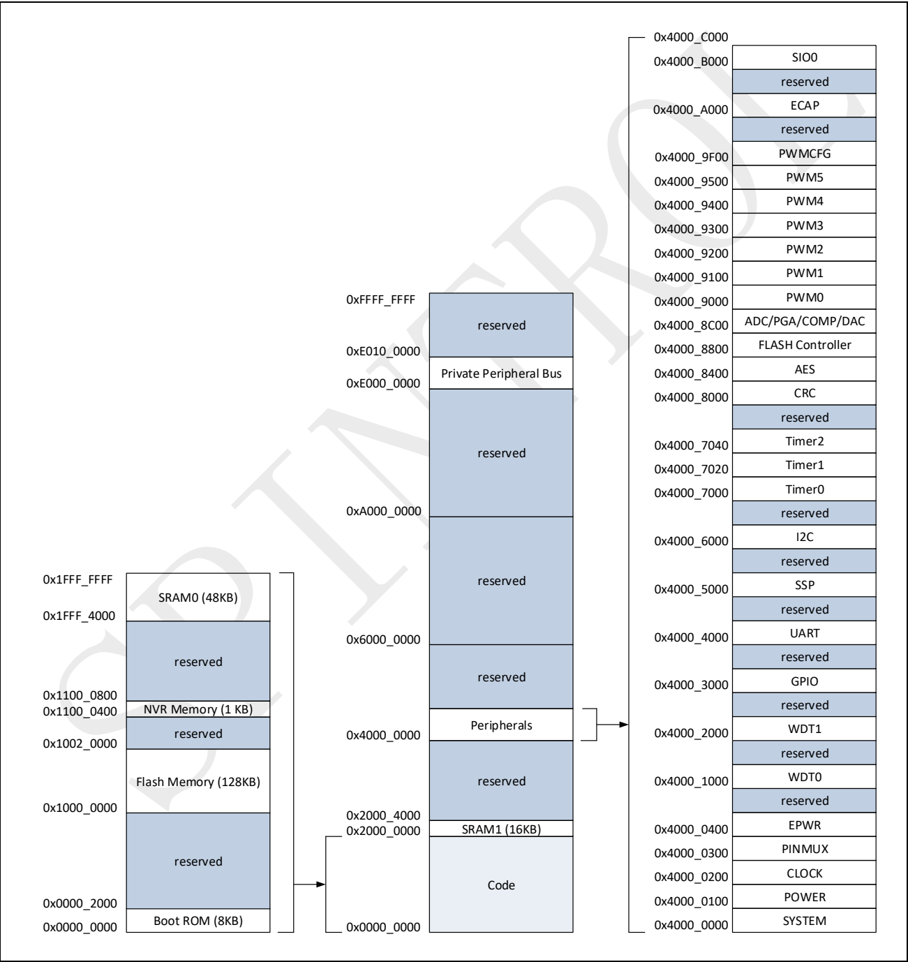
图 1-4：SPD1188 存储器映射
