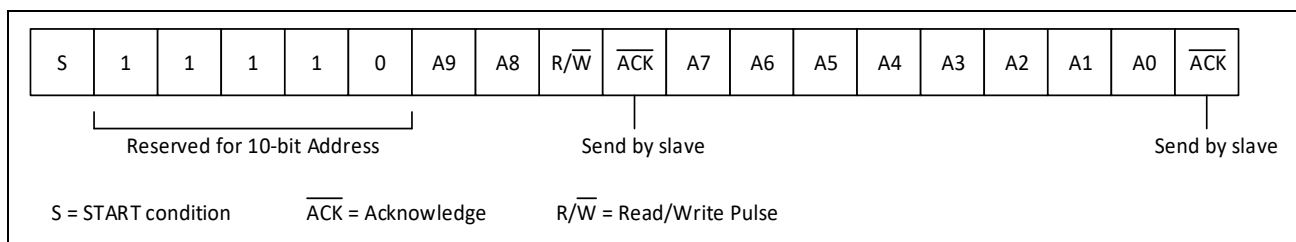
图 18-4: 10 位地址格式
