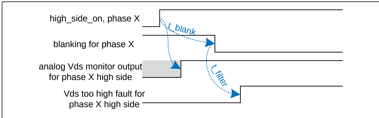
图 26-6：故障信号的消隐和滤波效果
