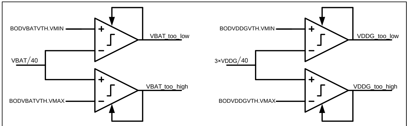
图 26-4: VBAT 和 VDDG 电源检测器
