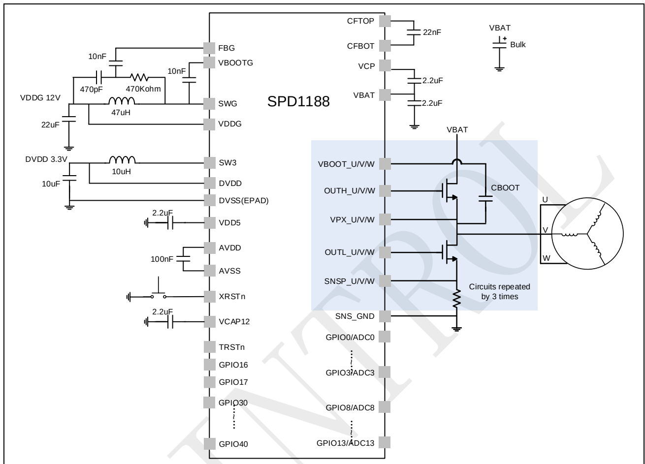
图 1-2: 典型应用图
