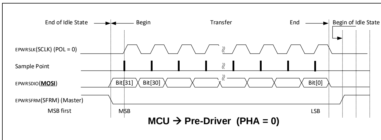
图 24-2: MCU 向高压模块发送数据
