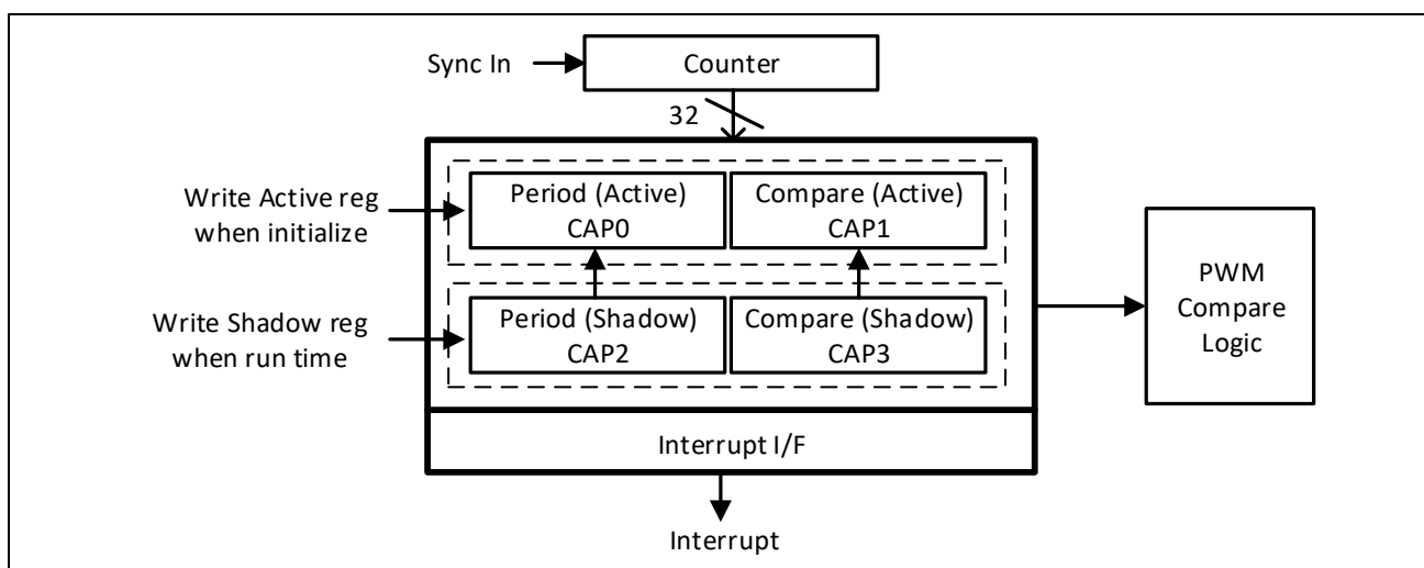
图 11-9：APWM 模式下 PRD 和 CMP 的有效值和影子值
