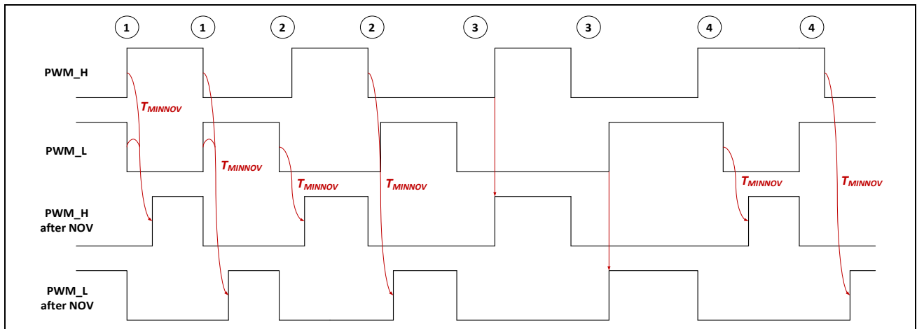
图 26-3: NOV 模块工作描述
