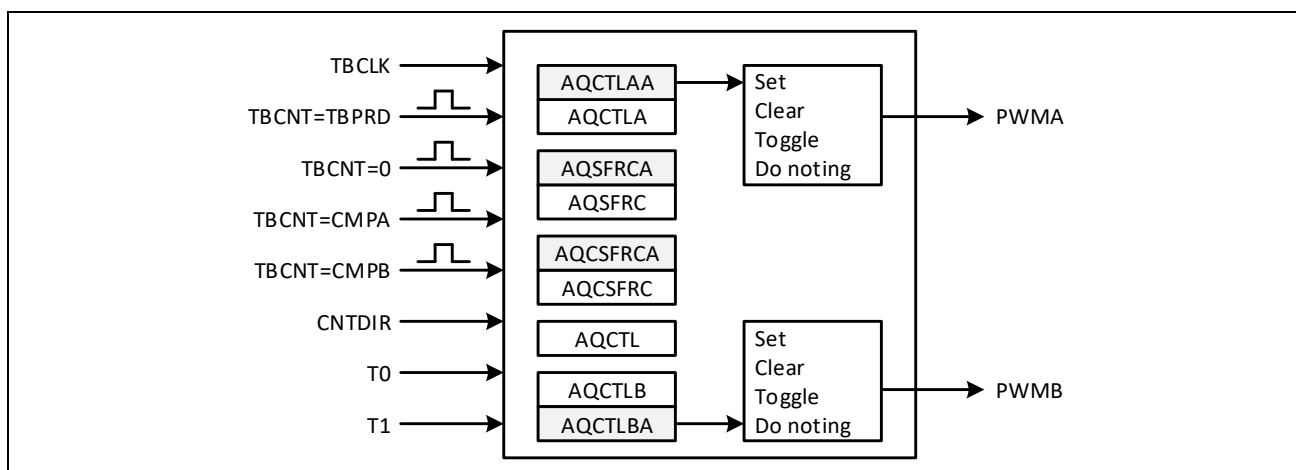
图 10-8：行为限定子模块输入输出
