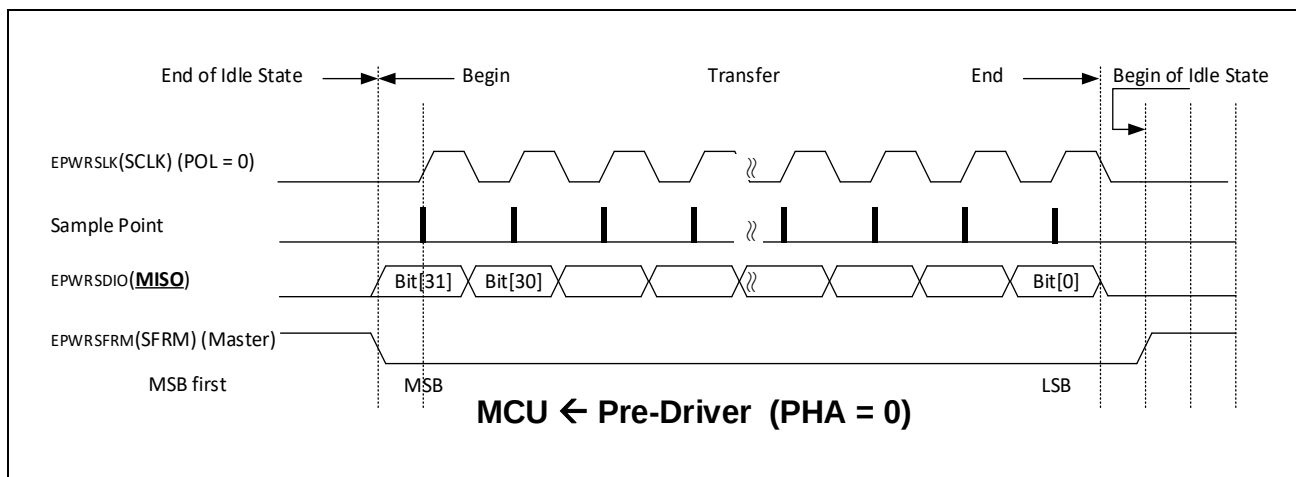
图 24-3: MCU 从高压模块接受数据
